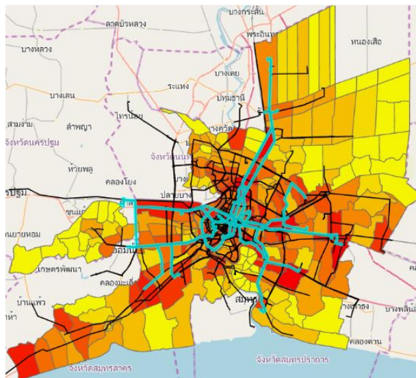
รูปที่ 6: เส้นทางรถโดยสารประจำทางที่จะทำการย้ายไปให้บริการในเขตพื้นที่ยังไม่มีบริการสาธารณะ
