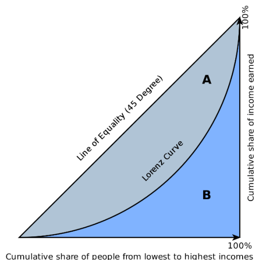
รูปที่ 5: การหาค่าสัมประสิทธิ์จีนิ Gini = A / (A+B)
